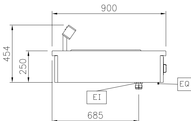
Zij aanzicht
